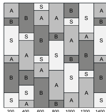
RADIATORE RIFLESSI H1400
